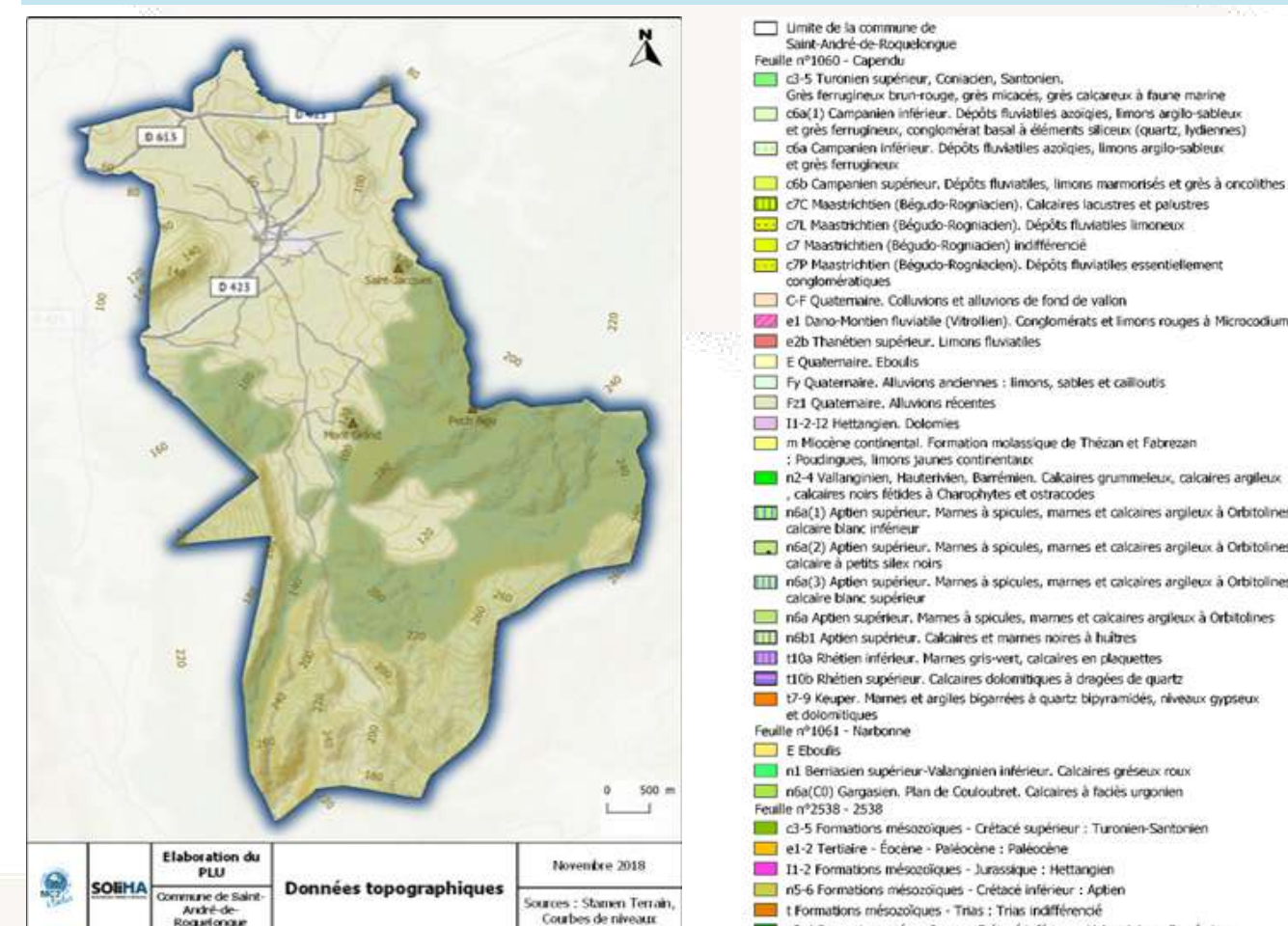
Carte 22 : Relief de la commune de Saint-André-de-Roquelongue
