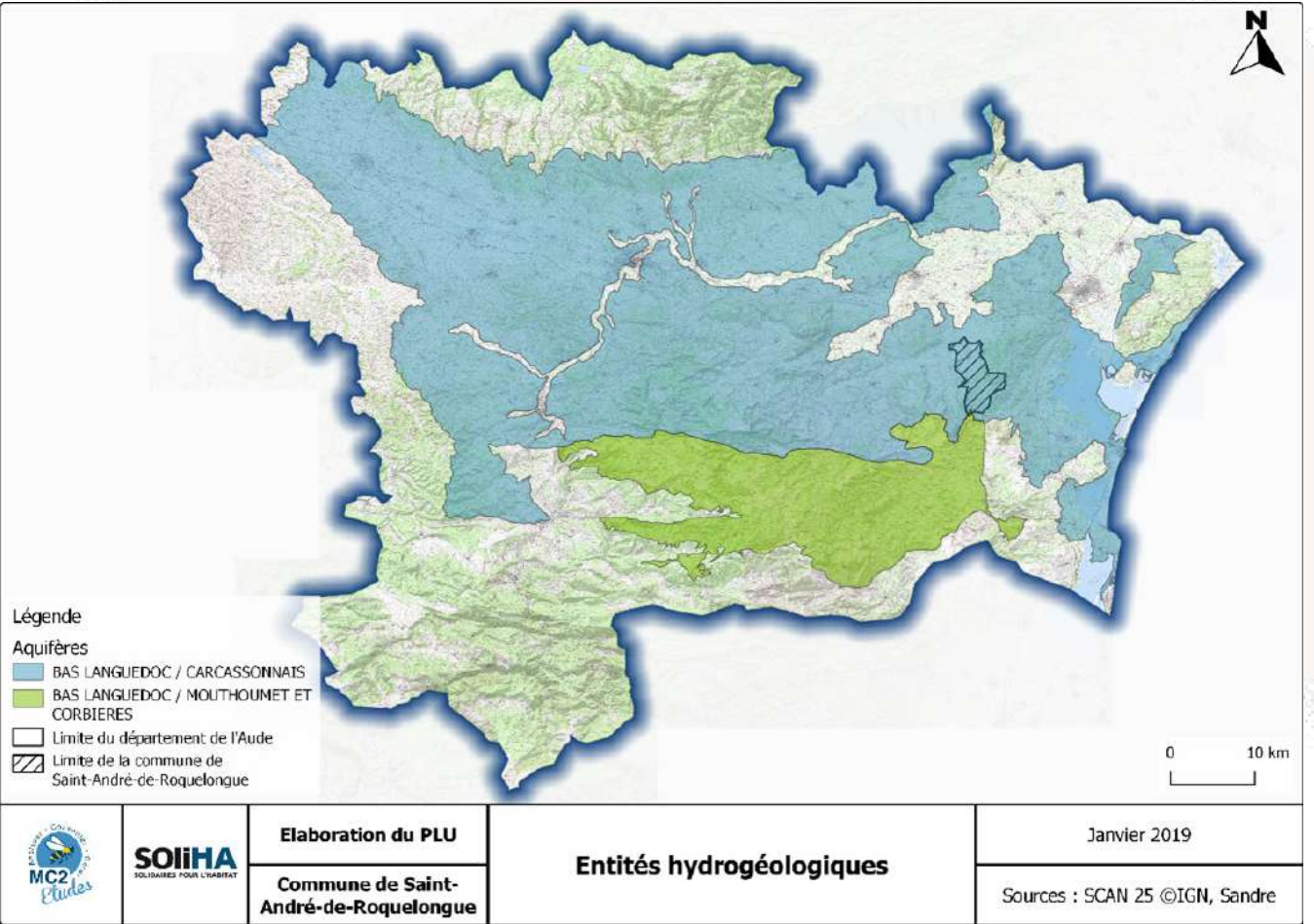
Carte 25 : Entités hydrogéologiques sur la commune
